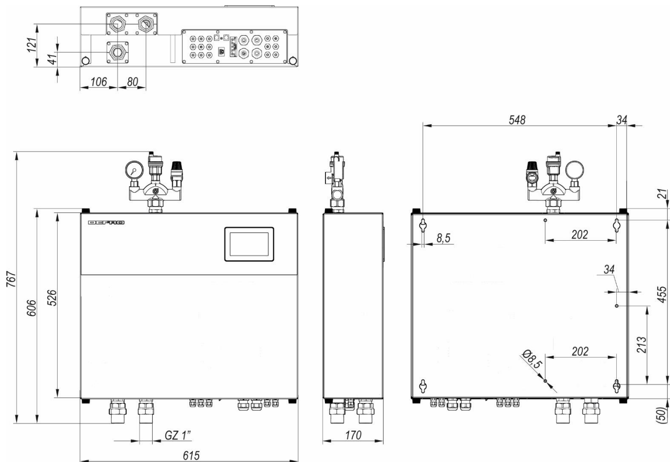
Rysunek 7. Wymiary hydromodułu pompy ciepła DHPI MONOTEC.
