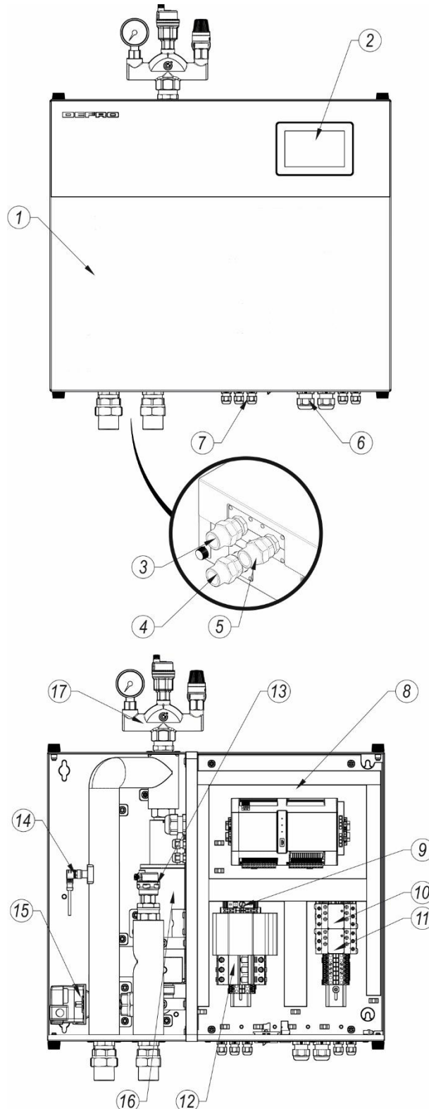
Rysunek 4. Budowa skrzynki instalacyjnej.
