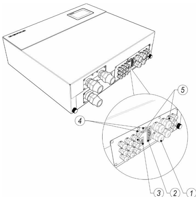
Rysunek 15. Opis złączy elektrycznych.
