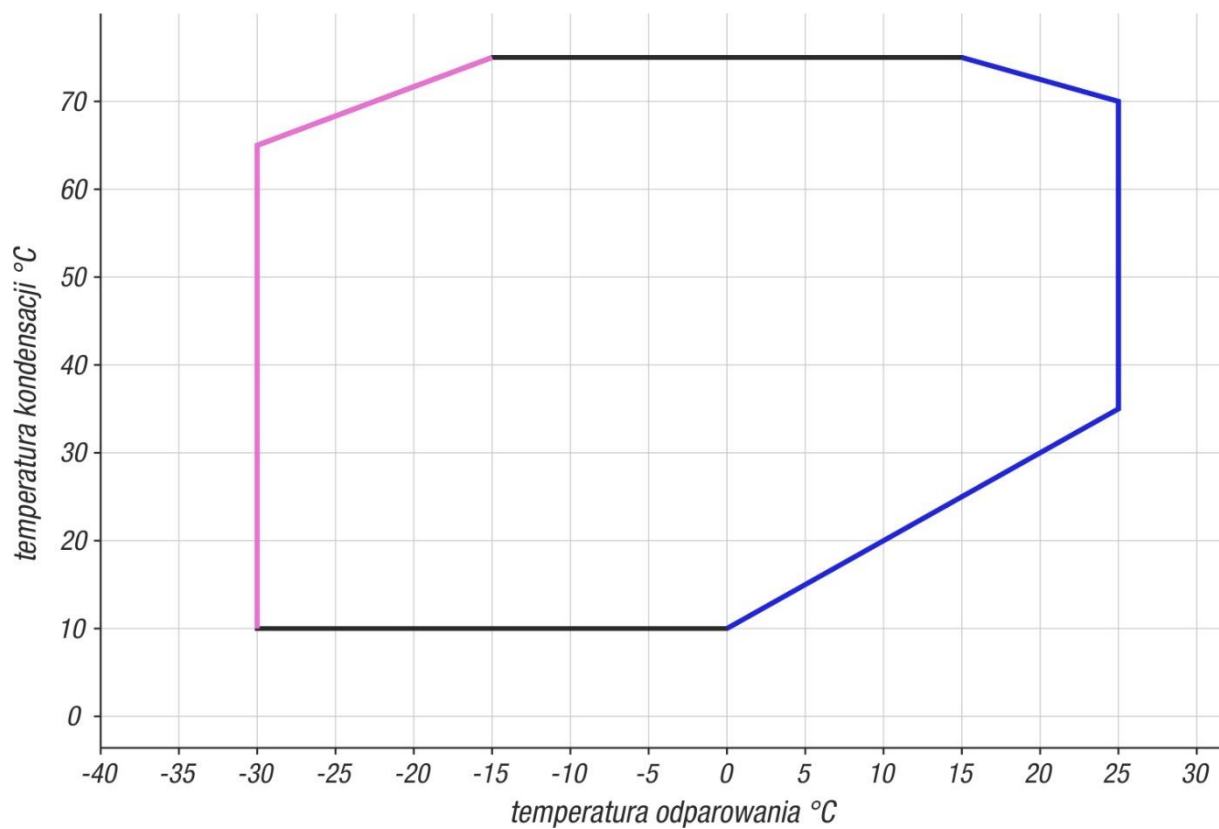
Rysunek 8. Koperta pracy sprężarki pompy ciepła DHPI MONOTEC
