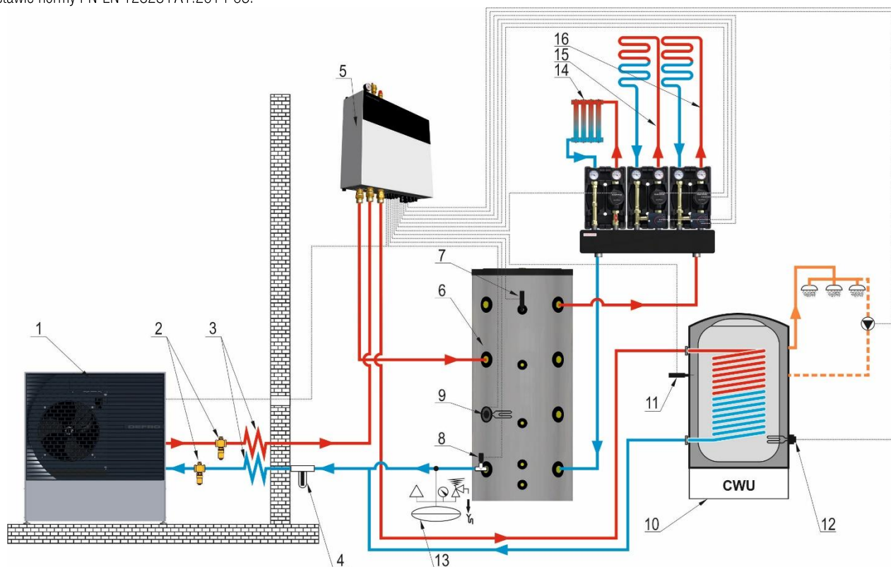
Rysunek 14. Przykładowy schemat instalacji grzewczej z pompą ciepła DHPi MONOTEC.
