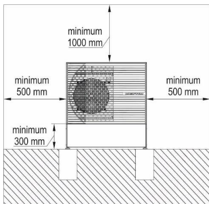
Rysunek 11. Miejsce montażu pompy ciepła rzut przodu.
