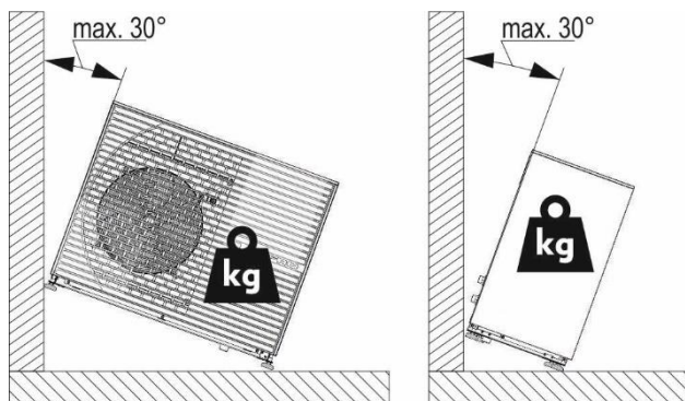
Rysunek 5. Maksymalne dopuszczalne przechylenie jednostki zewnętrznej.
