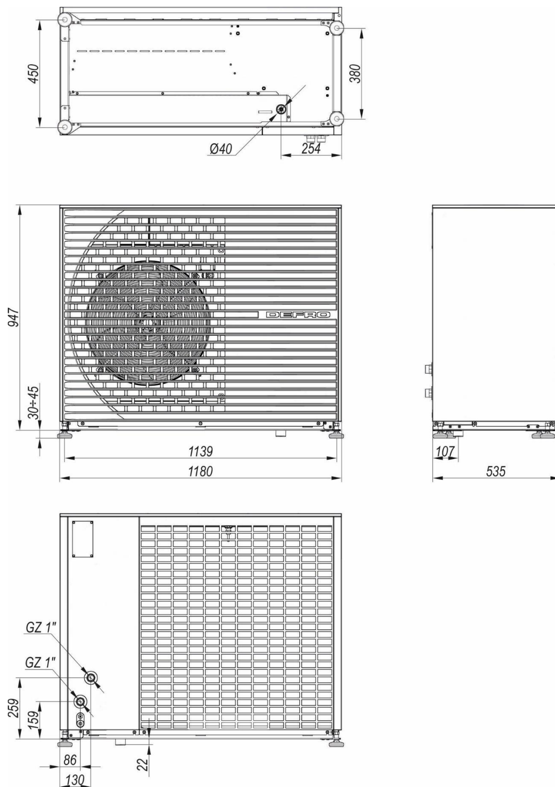
Rysunek 6. Wymiary pompy ciepła DHPi MONOTEC.
