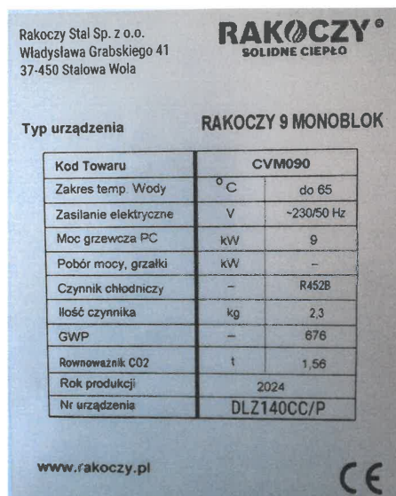
Heat pump Rakoczy 9 Monoblok – Unit label –
