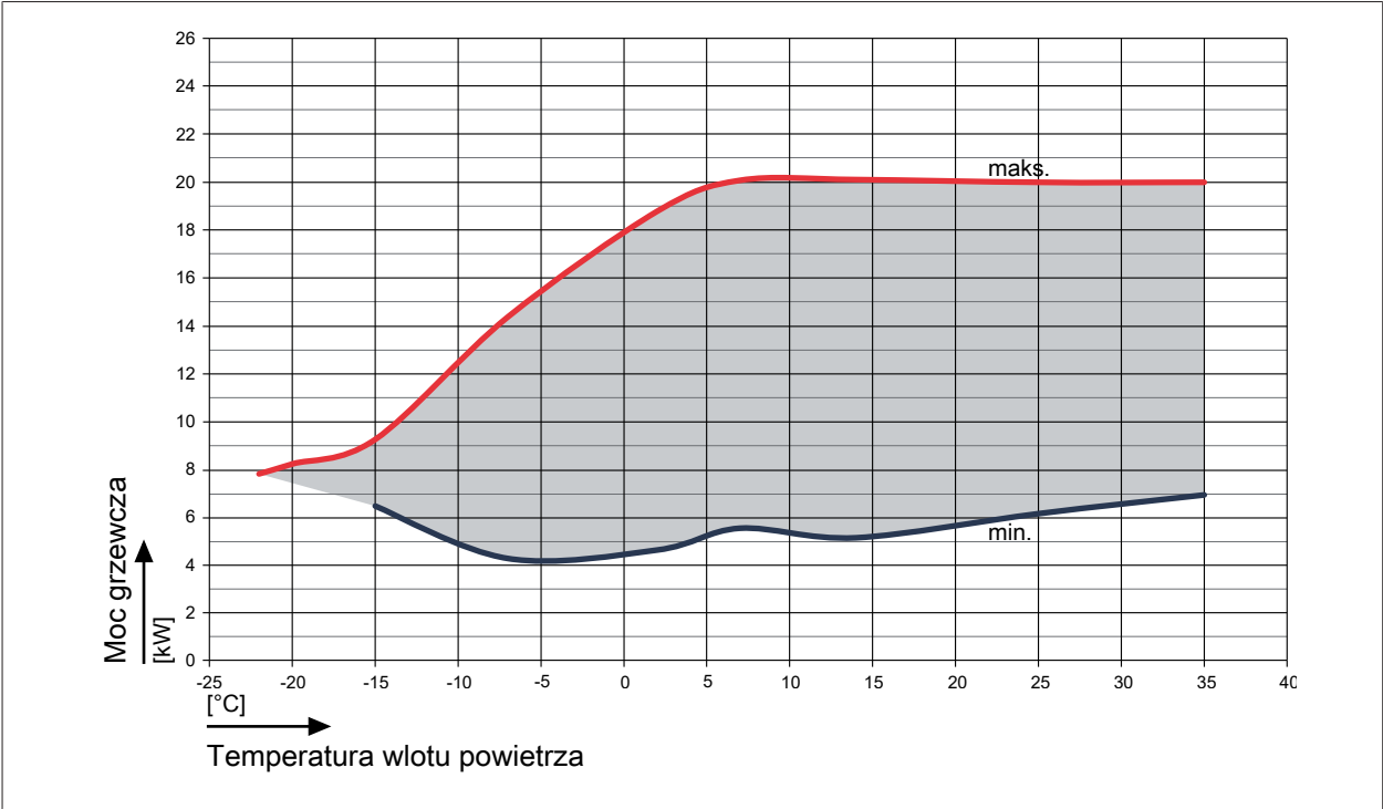
Rys. 8: Moc grzewcza CHA-16/20 przy zasilaniu 65°C
