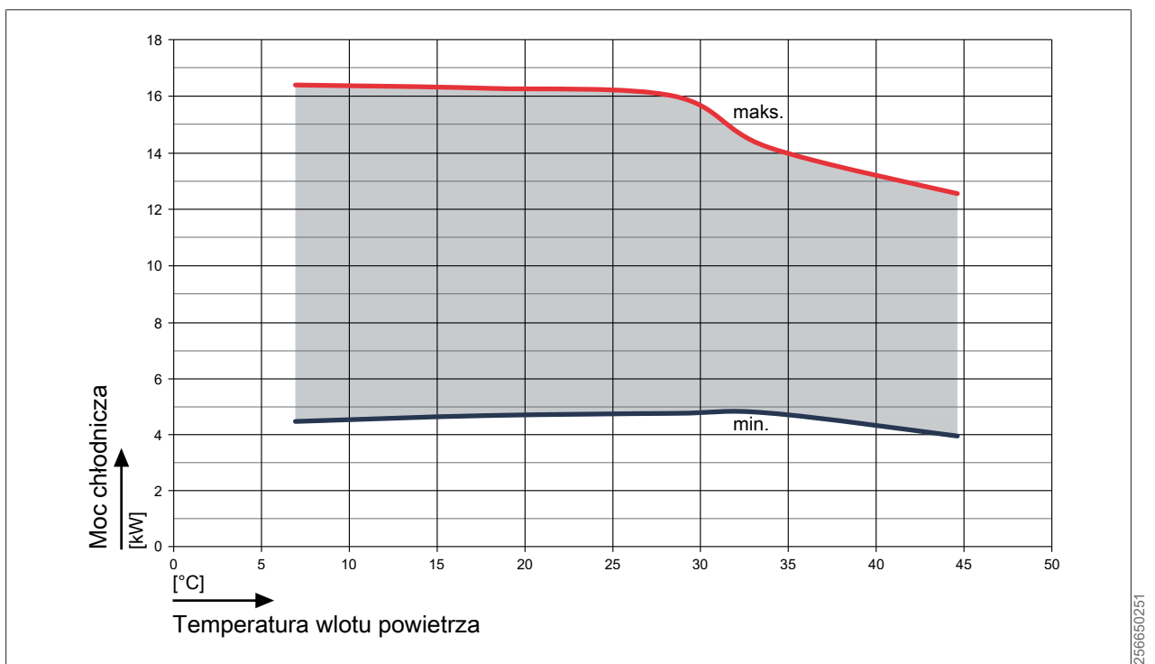
Rys. 10: Moc chłodnicza CHA-16/20 przy zasilaniu 7°C
