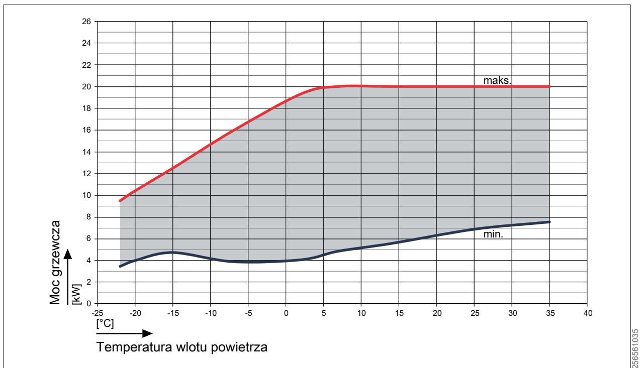
Rys. 7: Moc grzewcza CHA-16/20 przy zasilaniu 55°C
