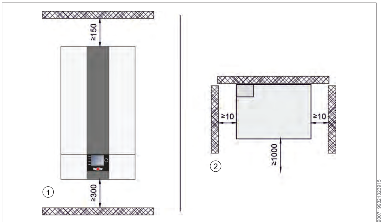
1 Widok z przodu IDU
