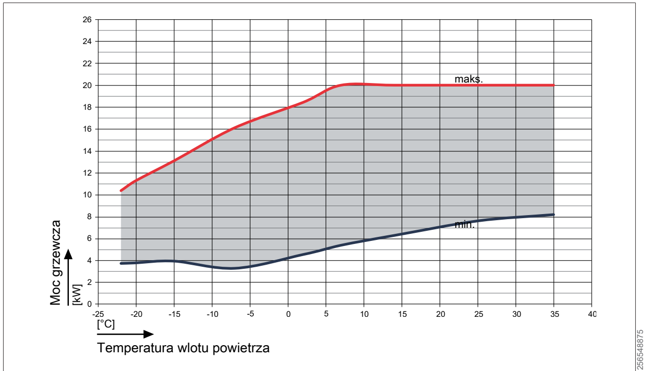
Rys. 6: Moc grzewcza CHA-16/20 przy zasilaniu 45°C
