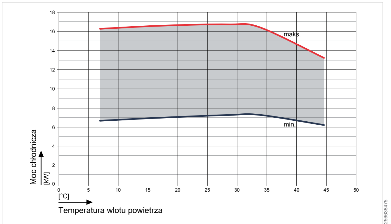
Rys. 9: Moc chłodnicza CHA-16/20 przy zasilaniu 18°C
