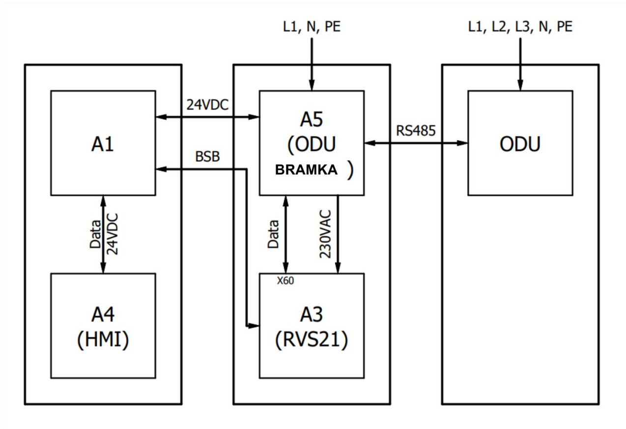
Schemat połączeń bramek ODU (A5)
